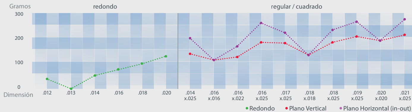
Fuerza de recuperación media con una desviación de 2 mm sobre una distancia de 12 mm
